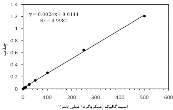
شکل 2- منحنی استاندارد گالیک اسید جهت اندازه‌گیری فنول کل
