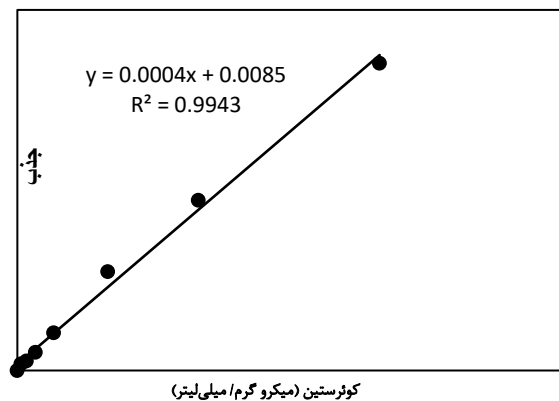
شکل 1- منحنی استاندارد کوئرستین جهت اندازه‌گیری فلاونوئید کل
