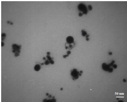
شکل 1. تصویر TEM از نانوذرات نقره بیوسنتزی از گیاه بومی زرین گیاه ( D. kotschy ).
