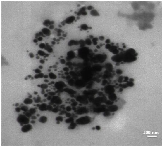
شکل ۱. تصویر TEM از نانوذرات نقره عمدتاً کروی زیست‌فرموله شده از گیاه سیاه‌دانه دشتی.
